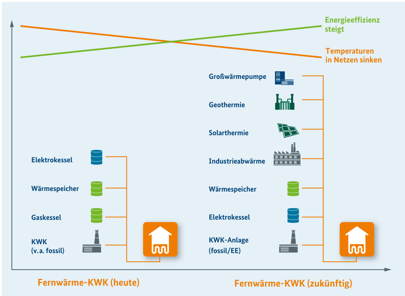
Abbildung 5: Modernisierung Fernwärme
